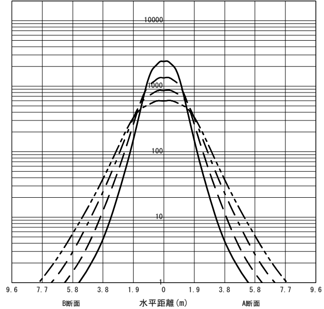
○直射水平面照度 (全光束 : 11100 × 1 = 11100lm/台) 照度 (lx) — H1.50m --- H2.00m - - - H2.50m - · - · H3.00m (保守率 : 1.00)
