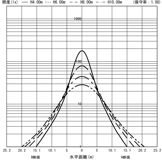
○直射水平面照度 (全光束: 9500 × 1 = 9500lm/台)
