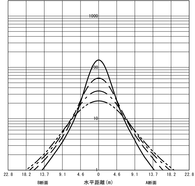
○直射水平面照度 (全光束: 7400 × 1 = 7400lm/台) 照度 (lx) — H4.00m --- H6.00m - - - H8.00m - · - · H10.00m (保守率: 1.00)
