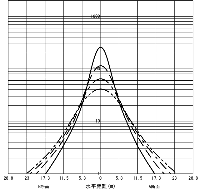
○直射水平面照度 (全光束: 13700 × 1 = 13700lm/台)
