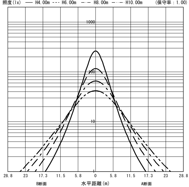
○直射水平面照度 (全光束: 15200 × 1 = 15200lm/台)
