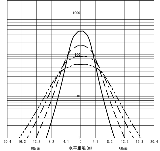
○直射水平面照度 (全光束: 12100 × 1 = 12100lm/台)
