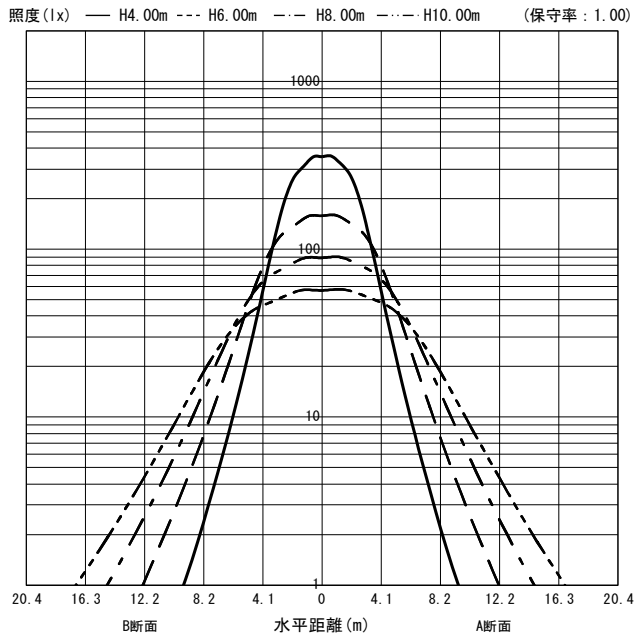
○直射水平面照度 (全光束 : 11800 × 1 = 11800lm/台)
