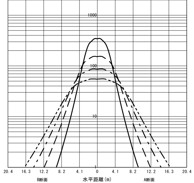
○直射水平面照度 (全光束 : 11400 × 1 = 11400lm/台) 照度 (lx) — H4.00m --- H6.00m - - - H8.00m - · - - H10.00m (保守率 : 1.00)
