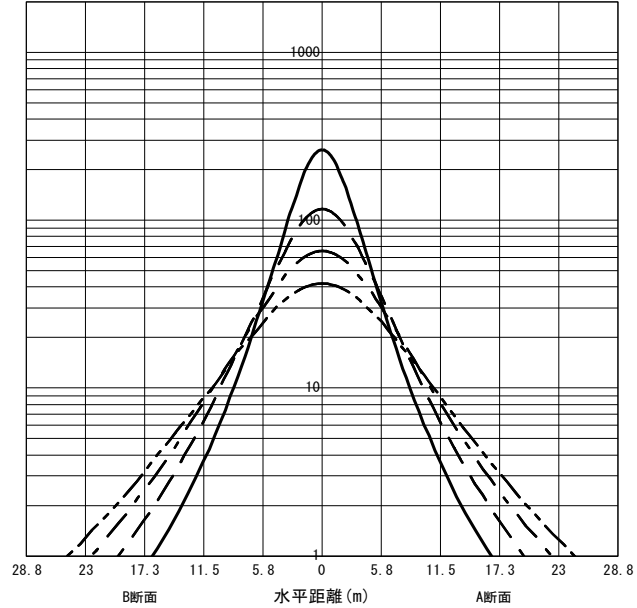
○直射水平面照度 (全光束: 15200 × 1 = 15200lm/台) 照度 (lx) — H4.00m --- H6.00m - - - H8.00m - · - · H10.00m (保守率: 1.00)
