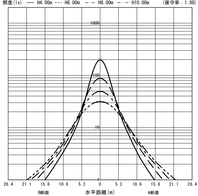
○直射水平面照度 (全光束: 10500 × 1 = 10500lm/台)
