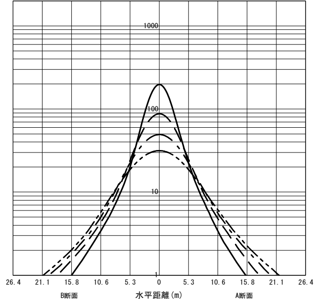
○直射水平面照度 (全光束: 10500 × 1 = 10500lm/台) 照度 (lx) — H4.00m --- H6.00m - - - H8.00m - · - · H10.00m (保守率: 1.00)
