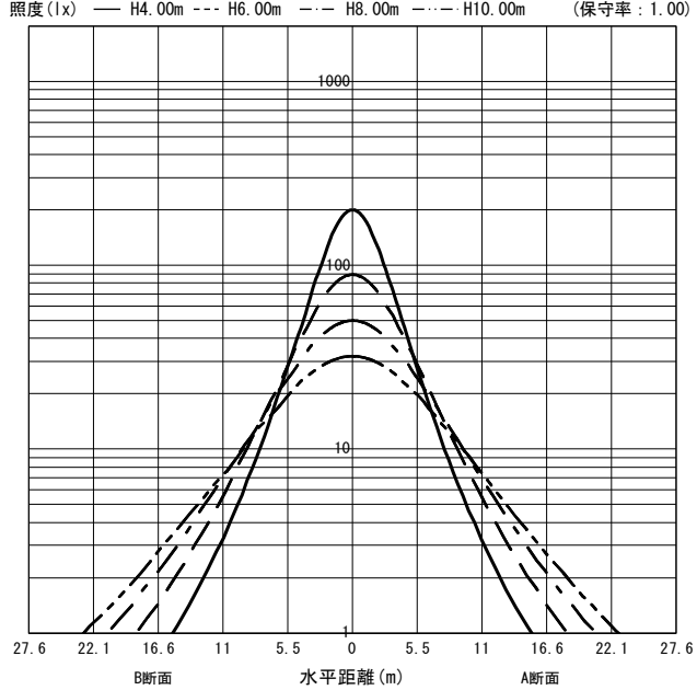
○直射水平面照度 (全光束: 11600 × 1 = 11600lm/台)
