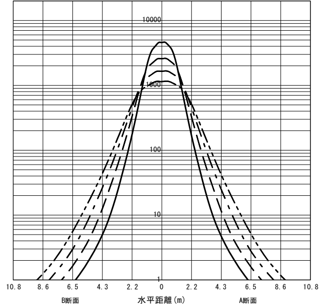
○直射水平面照度 (全光束 : 21300 × 1 = 21300lm/台) 照度 (lx) — H1.50m --- H2.00m - - - H2.50m - · - · H3.00m (保守率 : 1.00)
