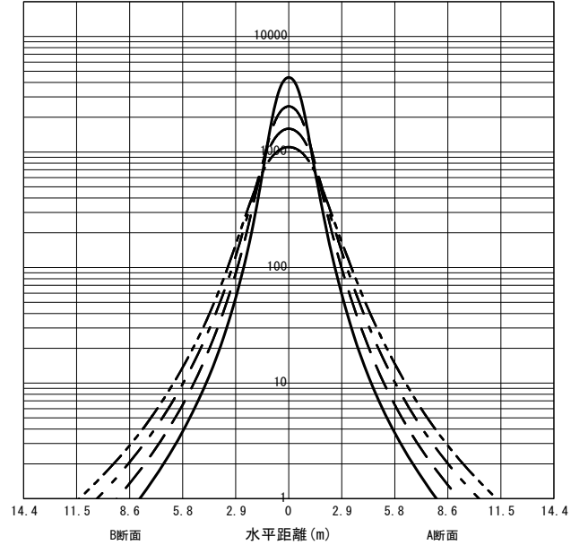
○直射水平面照度 (全光束: 18600 × 1 = 18600lm/台) 照度 (lx) — H1.50m --- H2.00m - - - H2.50m - · - · H3.00m (保守率: 1.00)
