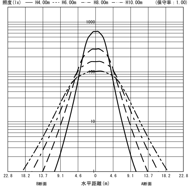
○直射水平面照度 (全光束 : 21300 × 1 = 21300lm/台)
