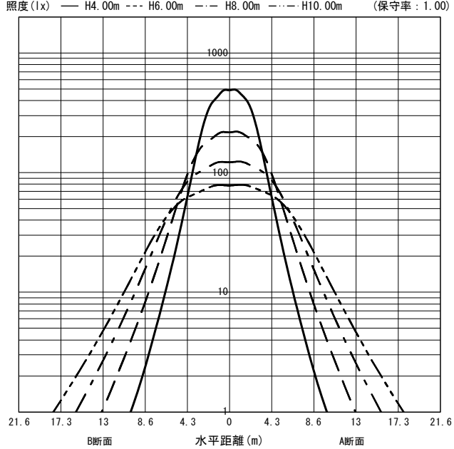
○直射水平面照度 (全光束 : 16200 × 1 = 16200lm/台)
