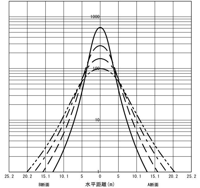
○直射水平面照度 (全光束: 18600 × 1 = 18600lm/台) 照度 (lx) — H4.00m --- H6.00m - - - H8.00m - · - · H10.00m (保守率: 1.00)
