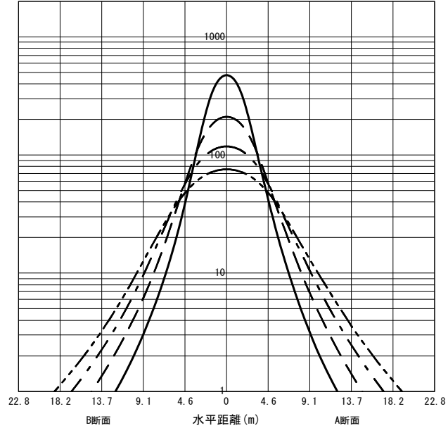
○直射水平面照度 (全光束 : 14200 × 1 = 14200lm/台) 照度 (lx) — H4.00m --- H6.00m - - - H8.00m - · - · H10.00m (保守率 : 1.00)
