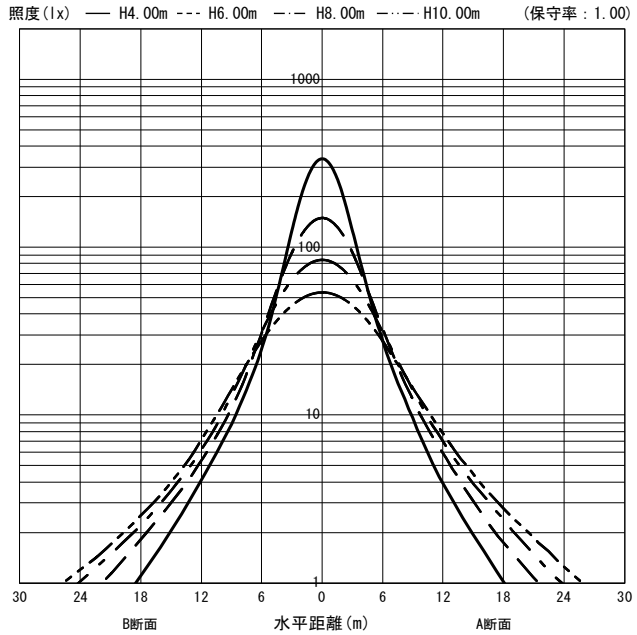
○直射水平面照度 (全光束 : 17900 × 1 = 17900lm/台)
