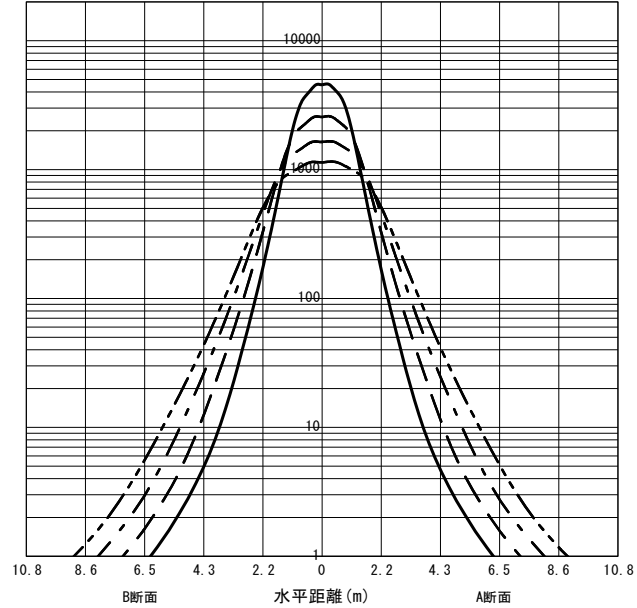
○直射水平面照度 (全光束 : 21200 × 1 = 21200lm/台) 照度 (lx) — H1.50m --- H2.00m - - - H2.50m - · - · H3.00m (保守率 : 1.00)
