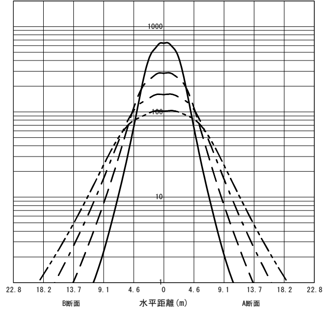
○直射水平面照度 (全光束: 21200 × 1 = 21200lm/台) 照度 (lx) — H4.00m --- H6.00m - - - H8.00m - · - · H10.00m (保守率: 1.00)
