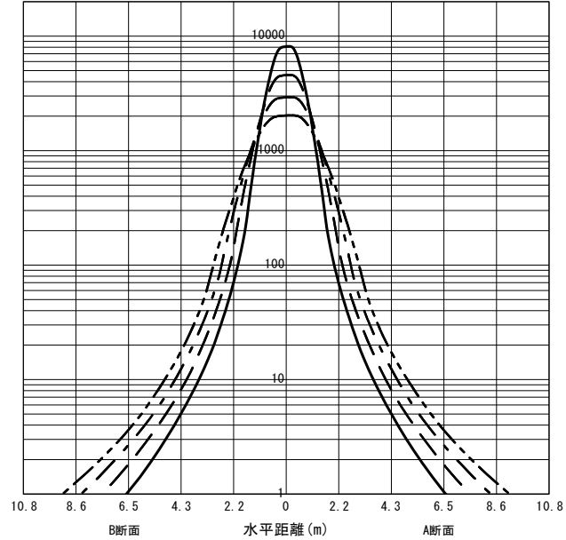
○直射水平面照度 (全光束 : 20500 × 1 = 20500lm/台) 照度 (lx) — H1.50m --- H2.00m - - - H2.50m - · - · H3.00m (保守率 : 1.00)
