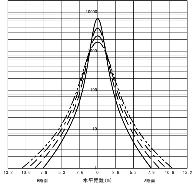
○直射水平面照度 (全光束: 18200 × 1 = 18200lm/台) 照度 (lx) — H1.50m --- H2.00m - - - H2.50m - · - · H3.00m (保守率: 1.00)
