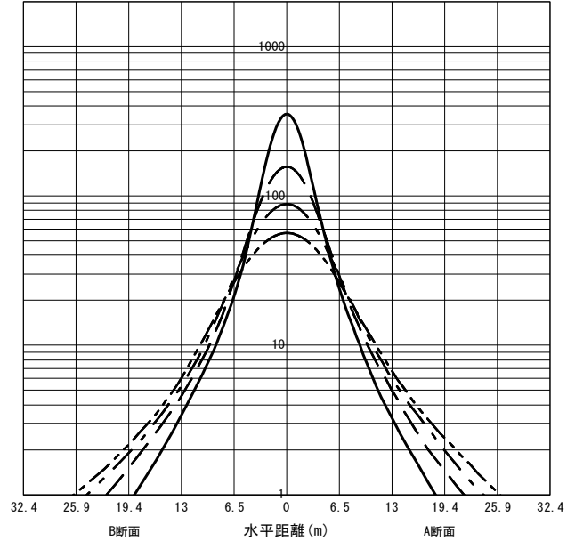
○直射水平面照度 (全光束: 18800 × 1 = 18800lm/台)
