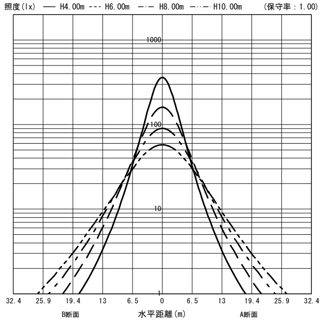
○直射水平面照度 (全光束 : 20900 × 1 = 20900lm/台)
