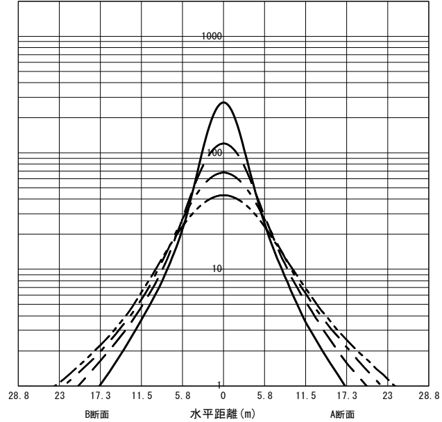
○直射水平面照度 (全光束: 14400 × 1 = 14400lm/台) 照度 (lx) — H4.00m --- H6.00m - - - H8.00m - · - · H10.00m (保守率: 1.00)
