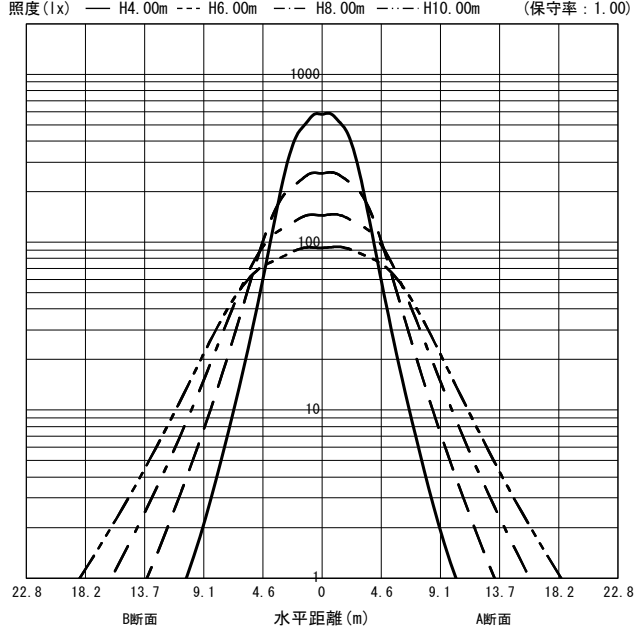
○直射水平面照度 (全光束 : 19200 × 1 = 19200lm/台)
