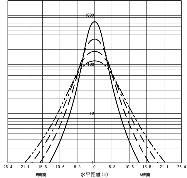
○直射水平面照度 (全光束: 22200 × 1 = 22200lm/台) 照度 (lx) — H4.00m --- H6.00m - - - H8.00m - · - · H10.00m (保守率: 1.00)
