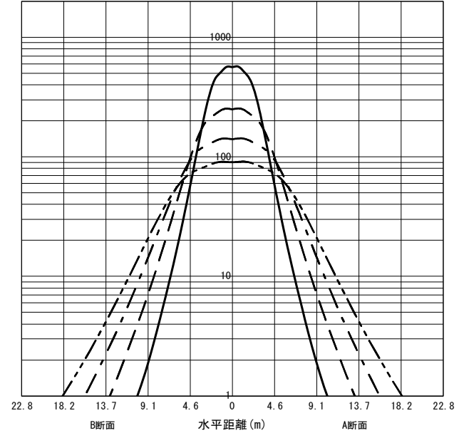
○直射水平面照度 (全光束: 18700 × 1 = 18700lm/台)
