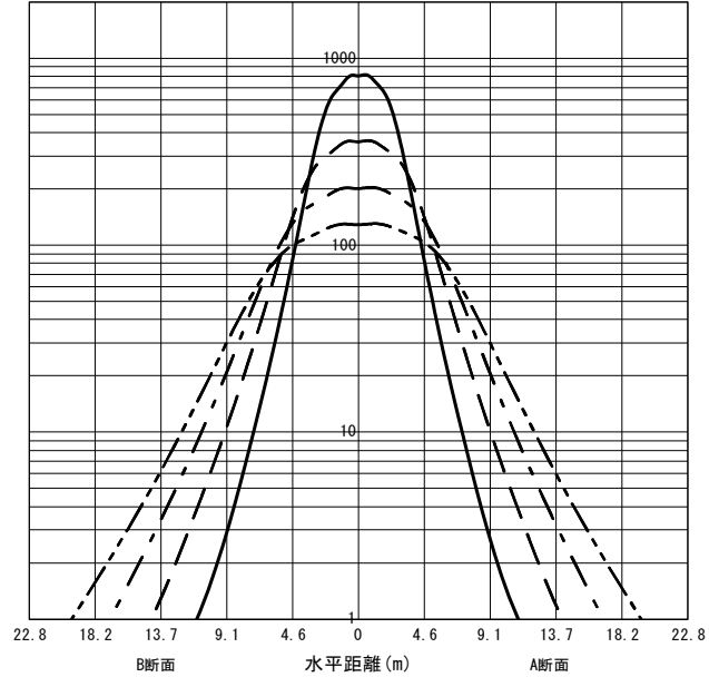
○直射水平面照度 (全光束 : 26700 × 1 = 26700lm/台) 照度 (lx) — H4.00m --- H6.00m - - - H8.00m - · - · H10.00m (保守率 : 1.00)
