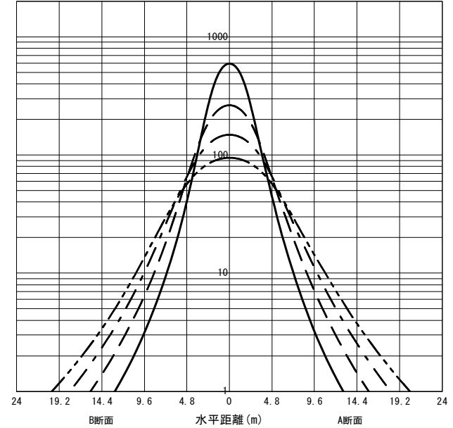
○直射水平面照度 (全光束 : 17800 × 1 = 17800lm/台)
