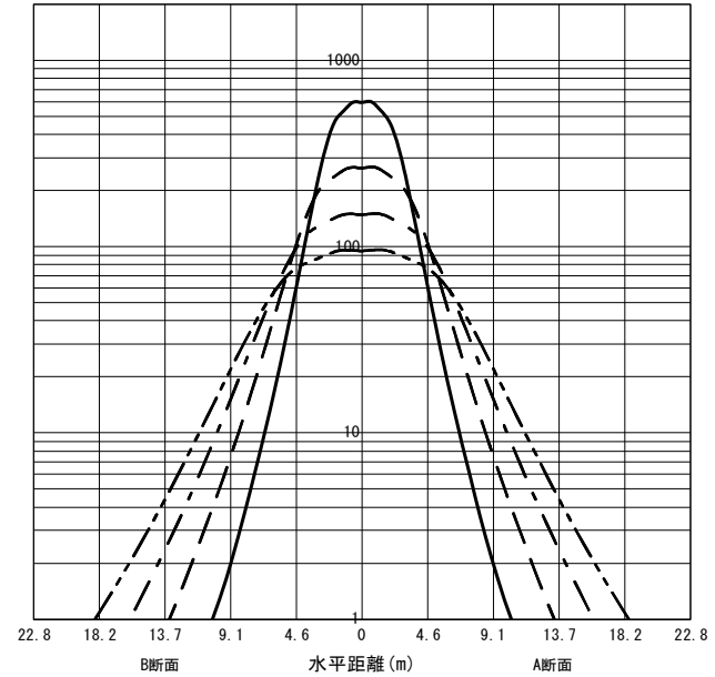
○直射水平面照度 (全光束: 19700 × 1 = 19700lm/台) 照度 (lx) — H4.00m --- H6.00m - - - H8.00m - · - · H10.00m (保守率: 1.00)
