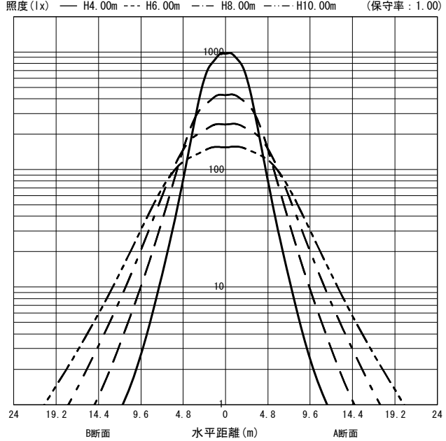
○直射水平面照度 (全光束 : 32100 × 1 = 32100lm/台)
