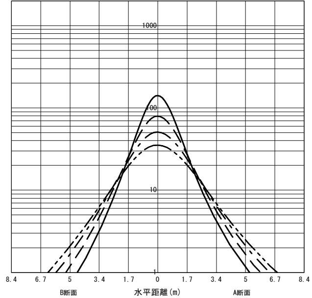
○直射水平面照度 (全光束: 1020 × 1 = 1020lm/台) 照度 (lx) — H1.50m --- H2.00m - - - H2.50m - · - · H3.00m (保守率: 1.00)
