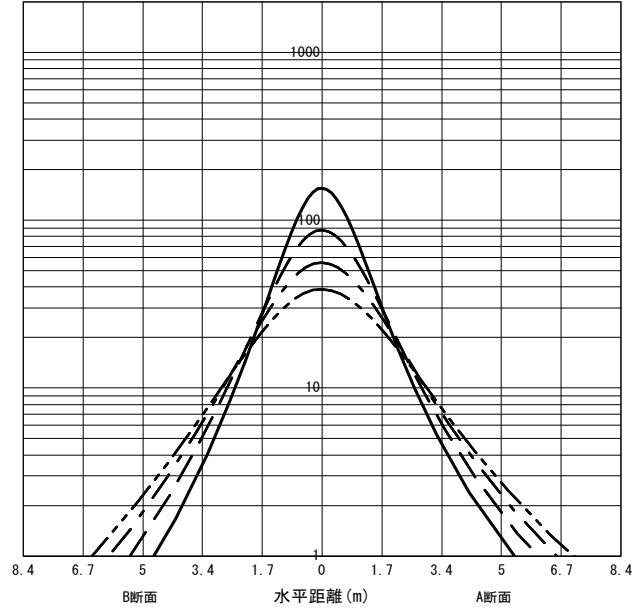
○直射水平面照度 (全光束: 1120 × 1 = 1120lm/台) 照度 (lx) — H1.50m --- H2.00m - - - H2.50m - · - · H3.00m (保守率: 1.00)
