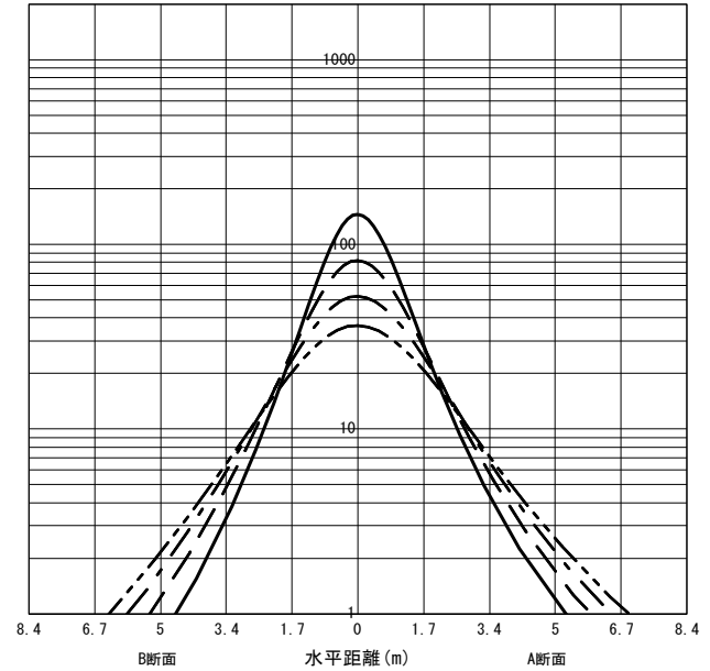
○直射水平面照度 (全光束: 1050 × 1 = 1050lm/台) 照度 (lx) — H1.50m --- H2.00m - - - H2.50m - · - · H3.00m (保守率: 1.00)
