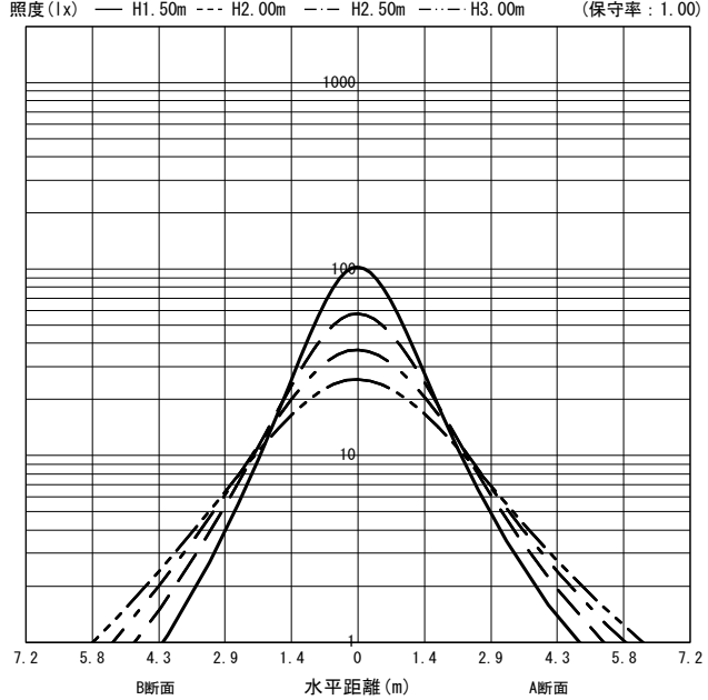
○直射水平面照度 (全光束 : 740 × 1 = 740lm/台)
