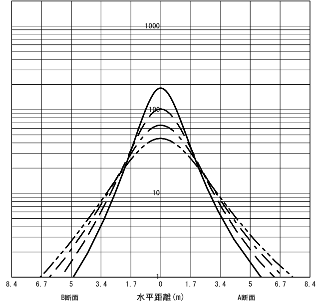
○直射水平面照度 (全光束: 1310 × 1 = 1310lm/台) 照度 (lx) — H1.50m --- H2.00m - - - H2.50m - · - · H3.00m (保守率: 1.00)
