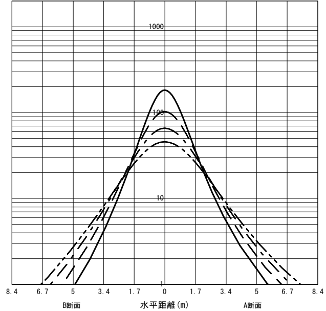
○直射水平面照度 (全光束: 1320 × 1 = 1320lm/台) 照度 (lx) — H1.50m --- H2.00m - - - H2.50m - · - · H3.00m (保守率: 1.00)
