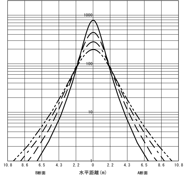
○直射水平面照度 (全光束 : 2400 × 3 = 7200lm/台) 照度 (lx) — H1.50m --- H2.00m - - - H2.50m - · - · H3.00m (保守率 : 1.00)
