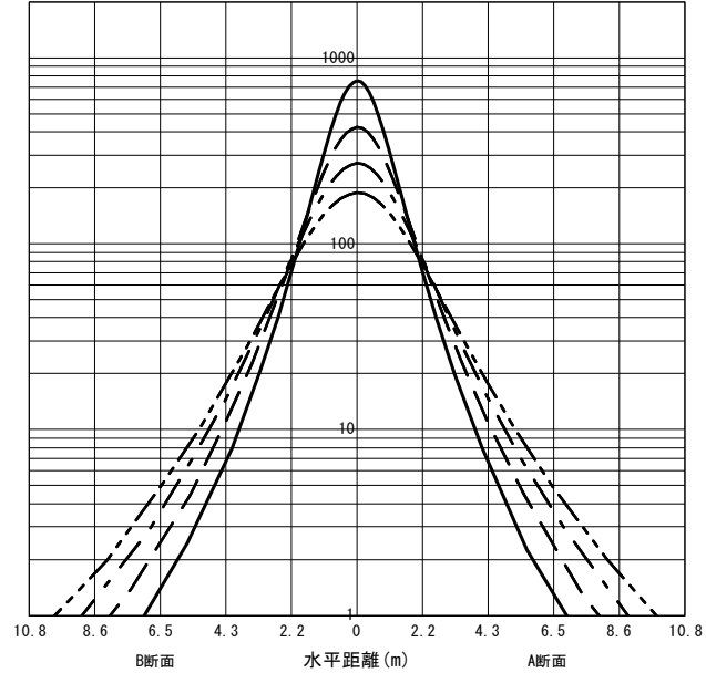
○直射水平面照度 (全光束: 2300 × 3 = 6900lm/台) 照度 (lx) — H1.50m --- H2.00m - - - H2.50m - · - · H3.00m (保守率: 1.00)
