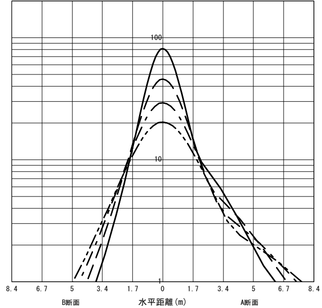
○直射水平面照度 (全光束: 1100 × 1 = 1100lm/台) 照度 (lx) — H1.50m --- H2.00m - - - H2.50m - · - · H3.00m (保守率: 1.00)
