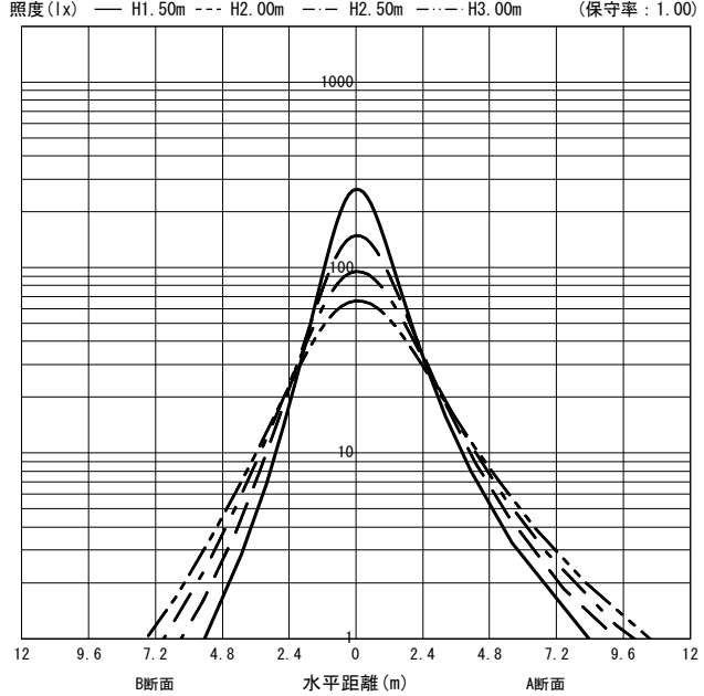
○直射水平面照度 (全光束: 3600 × 1 = 3600lm/台)
