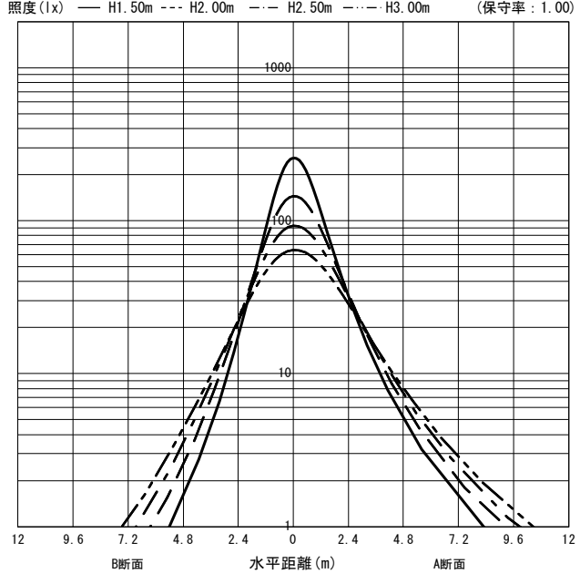
○直射水平面照度 (全光束: 3500 × 1 = 3500lm/台)
