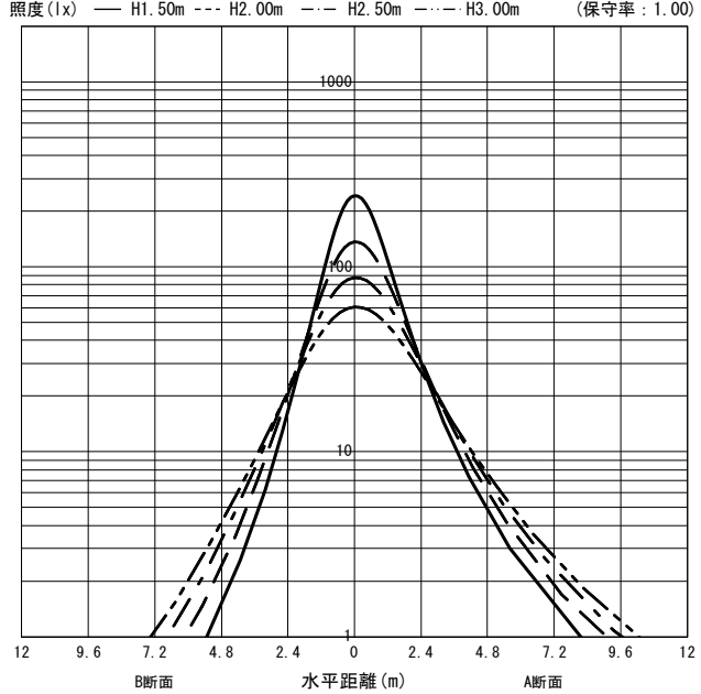
○直射水平面照度 (全光束: 3300 × 1 = 3300lm/台)
