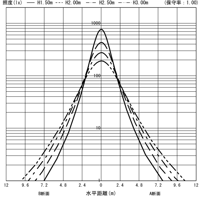
○直射水平面照度 (全光束: 2500 × 3 = 7500lm/台)
