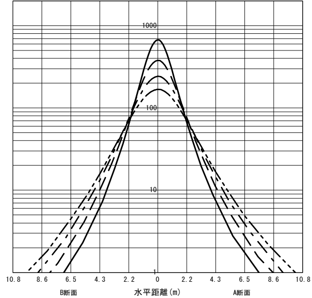
○直射水平面照度 (全光束: 2200 × 3 = 6600lm/台) 照度 (lx) — H1.50m --- H2.00m - - - H2.50m - · - · H3.00m (保守率: 1.00)
