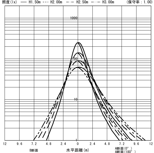
○直射水平面照度 (全光束: 1300 × 2 = 2600lm/台)
