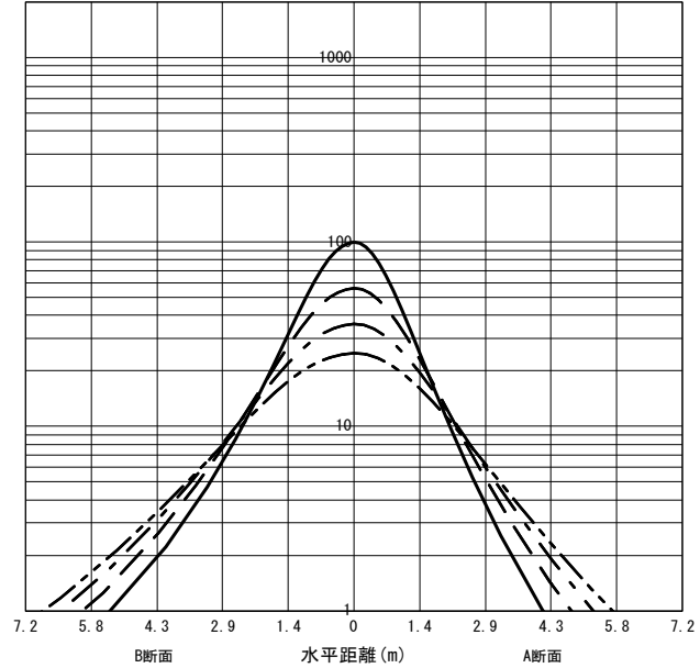
○直射水平面照度 (全光束: 980 × 1 = 980lm/台) 照度 (lx) — H1.50m --- H2.00m - - - H2.50m - · - · H3.00m (保守率: 1.00)
