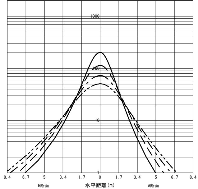
○直射水平面照度 (全光束 : 2000 × 1 = 2000lm/台) 照度 (lx) — H1.50m --- H2.00m - - - H2.50m - · - · H3.00m (保守率 : 1.00)
